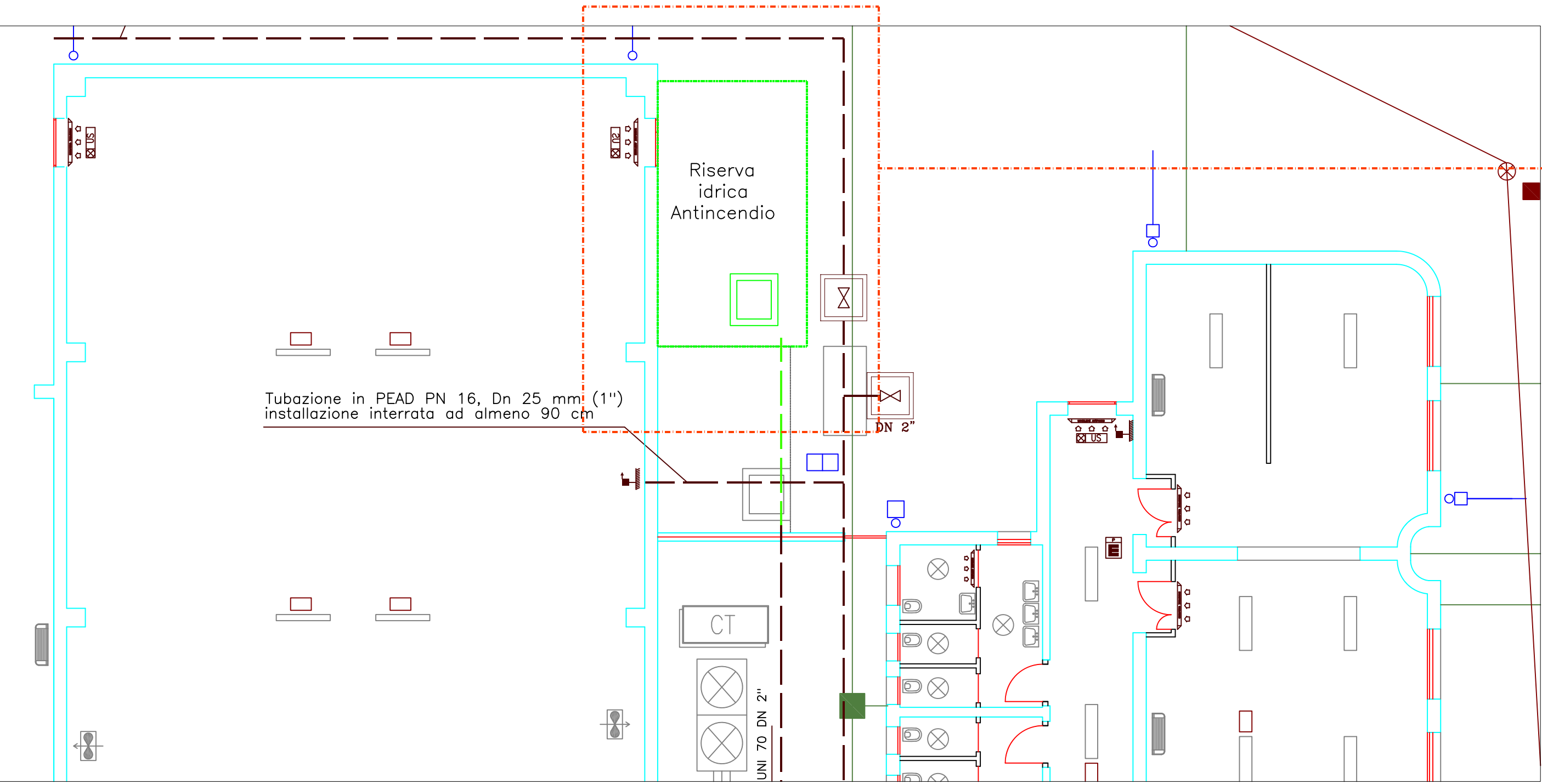
Particolare stato di progetto vasca antincendio scala 1:100
