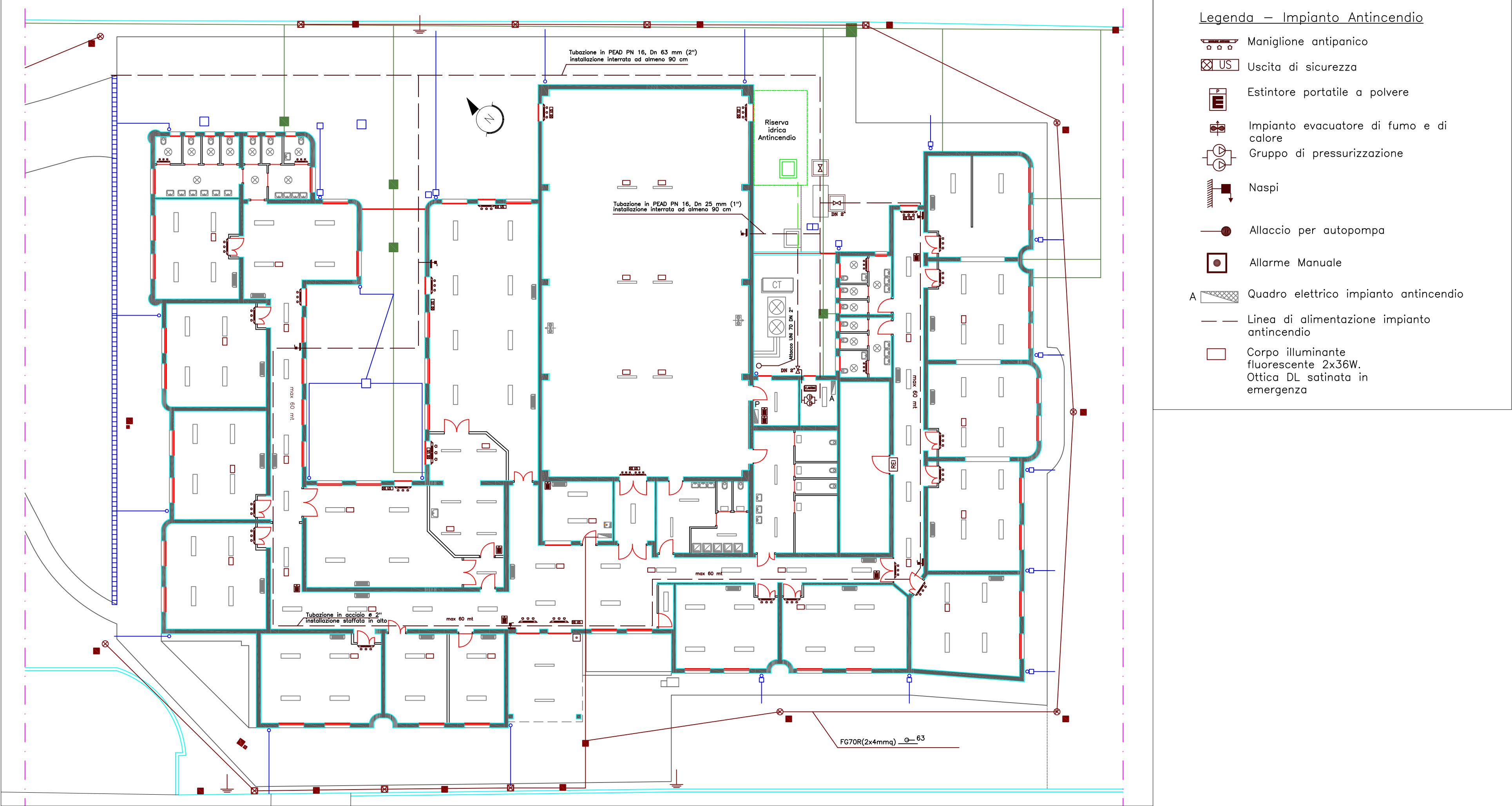
Pianta presidi antincendio stato attuale scala 1:200
