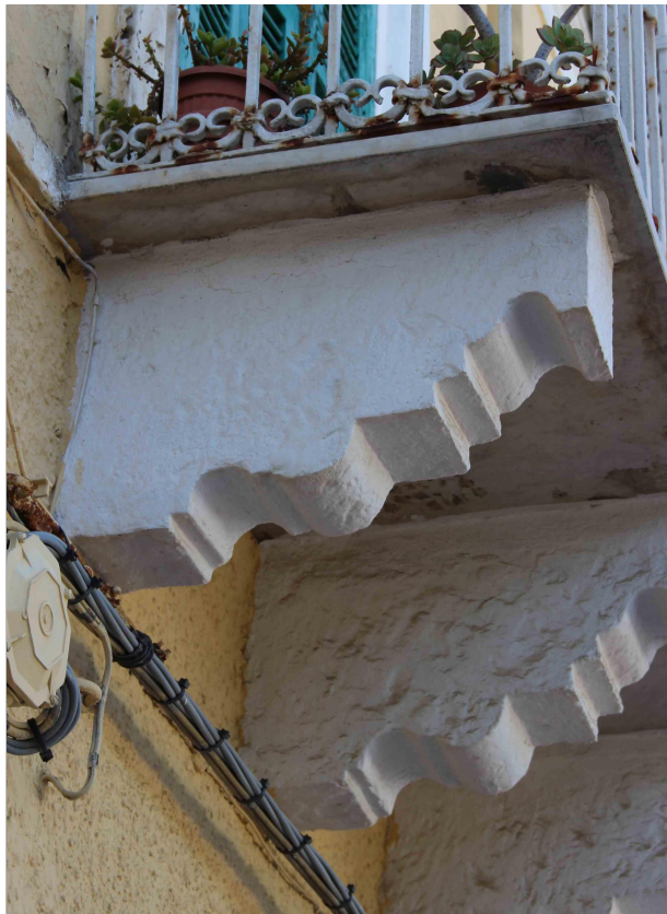
Mensola in pietra Questo tipo rappresenta una delle mensole più antiche, costituite da un unico blocco di pietra decorato.
